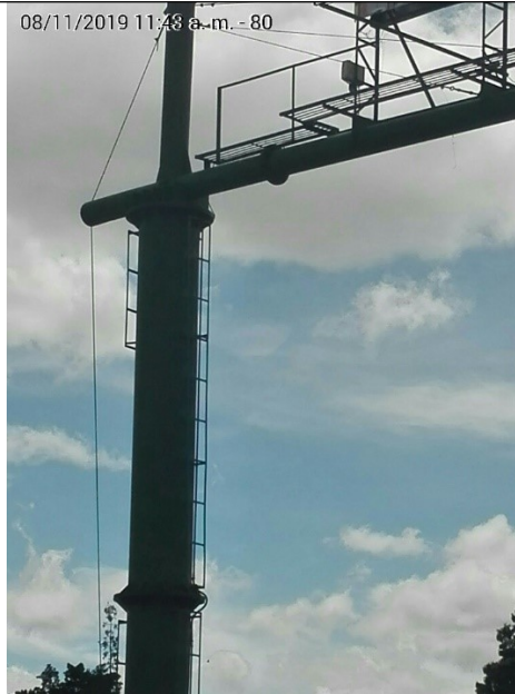
Foto No. 3: Detalles de la estructura y del mastil y tensores de la valla tubular, en buenas condiciones y estable, instalada en la Av. Carrera 68 No. 44-30 (dirección catastral), orientación Norte-Sur .
